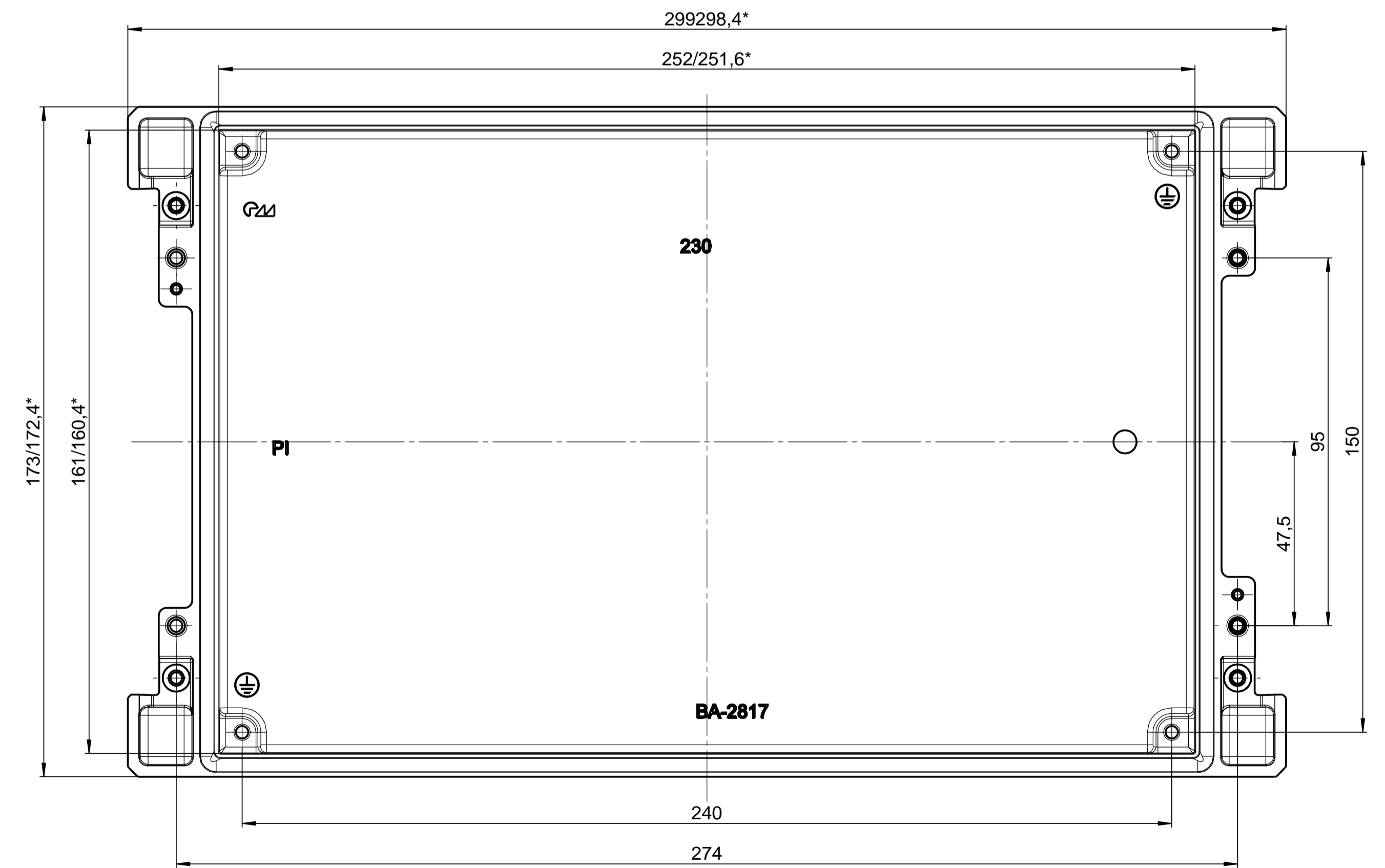
Deckel / lid
