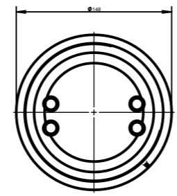
Deckel / Lid
