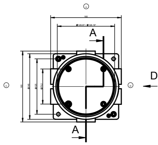
Unterteil / Base
