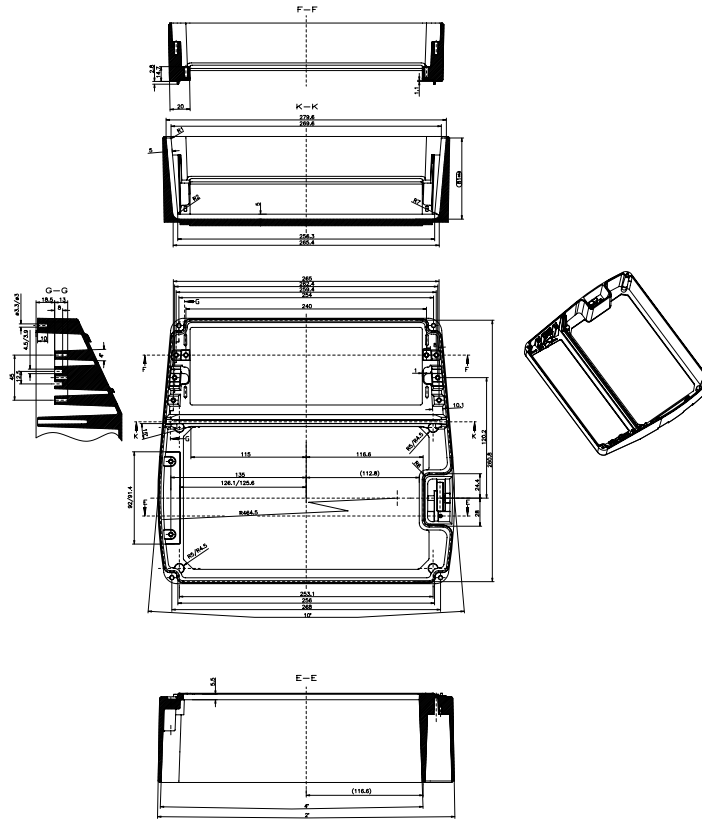
Abmessungen_Grundkörper_TF42_INNEN
